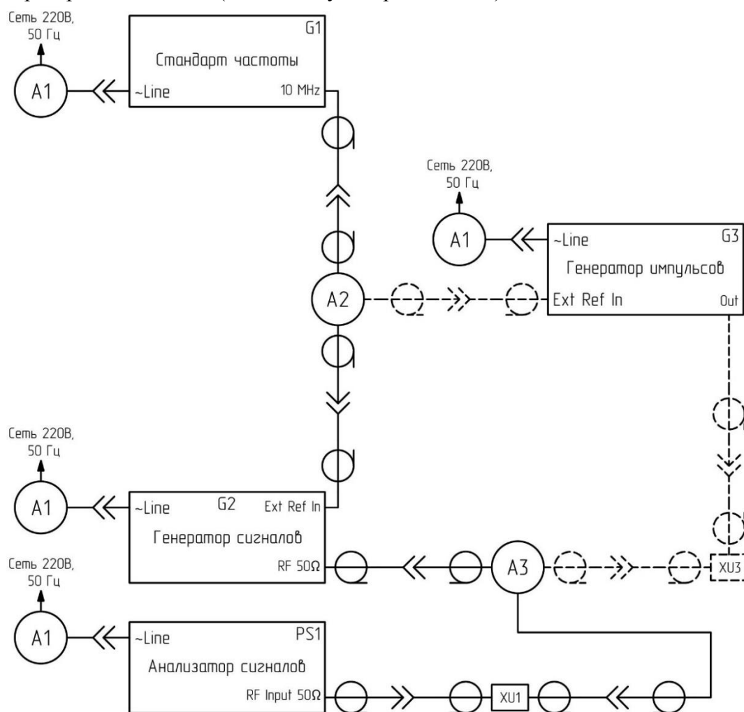
Рисунок 5 – Схема подключений для определения абсолютной погрешности измерений частоты входного синусоидального сигнала
