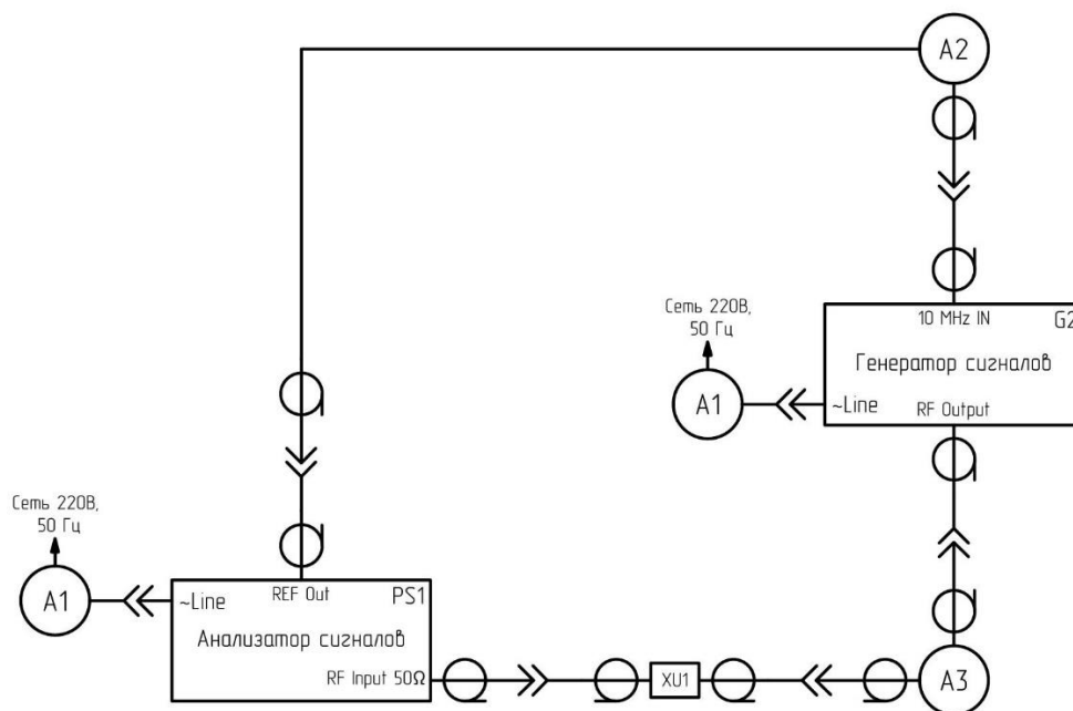
Рисунок 10 – Схема подключения для определения абсолютной погрешности измерений мощности на опорной частоте 100 МГц при изменении ослабления входного аттенюатора
