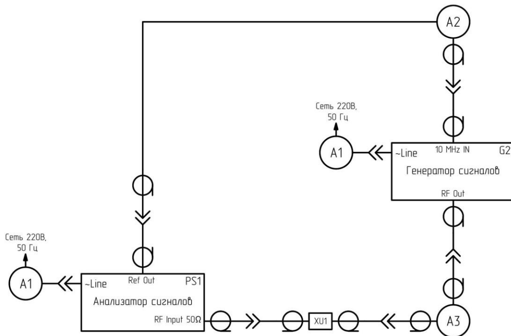
Рисунок 8 – Схема подключения для определения допускаемой погрешности установки номинальных значений полос пропускания по уровню минус 3 дБ
