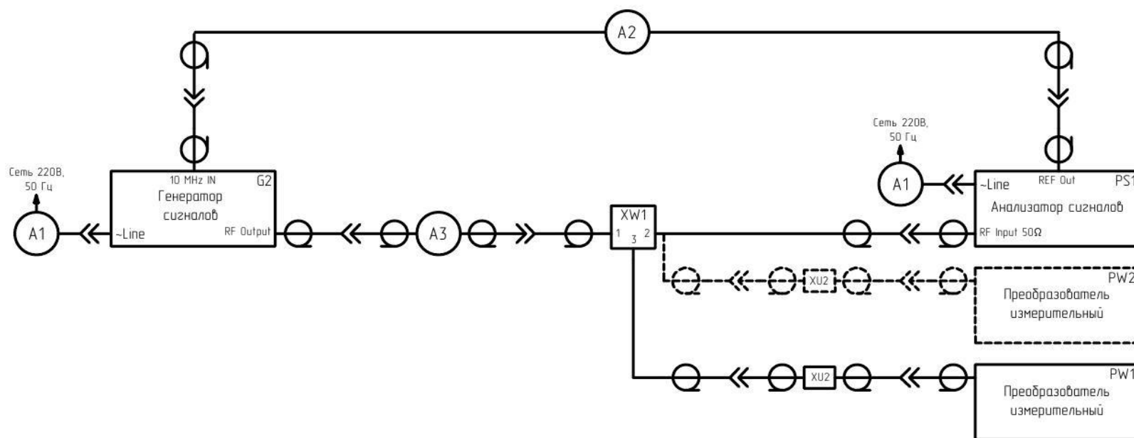
Рисунок 9 – Схема подключений для определения абсолютной погрешности измерений мощности при ослаблении входного аттенюатора 10 дБ в диапазоне мощностей от минус 20 до минус 10 дБ (1 мВт)
