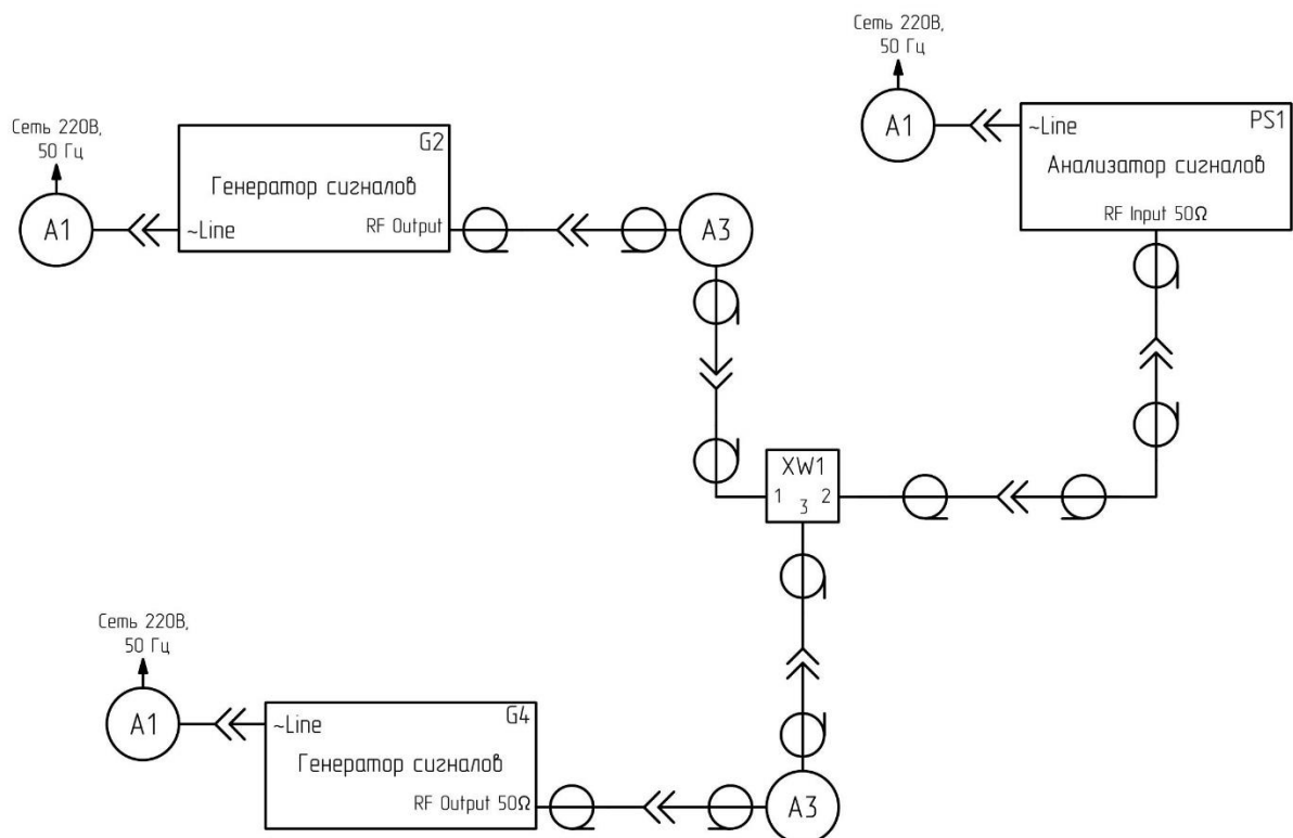
Рисунок 13 – Схема подключения для определения относительного уровня помех, обусловленных интермодуляционными искажениями третьего порядка, при ослаблении входного аттенюатора 10 дБ
